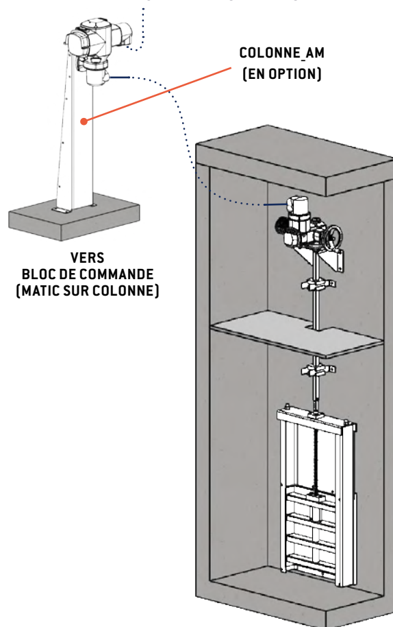
Exemple : Configuration pour vanne KSA 100-800
