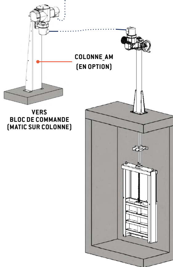
INSTALLATION DÉPORTÉE
