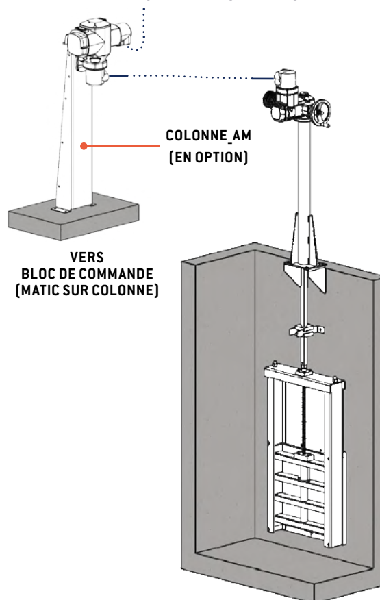
INSTALLATION DÉPORTÉE
